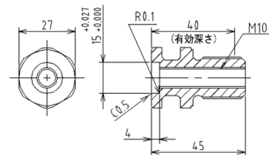
ジョイントピン詳細図
