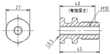
供試品取付ネジ詳細図 (ジョイントピンを除く)
